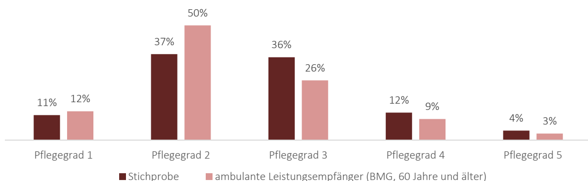
Abbildung 1: ZQP-Befragung pflegender Angehöriger in der COVID-19-Krise (n = 1.000); BMG (2020).
